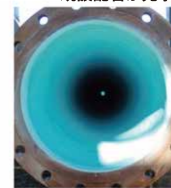
フレーク2層目塗布後、管内状況
