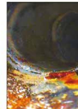
配管ジョイント部溶接不良
